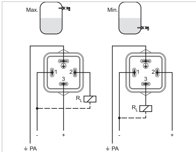
VEGASWING 51 con enchufe de válvula según DIN 4400
